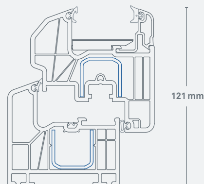
Prestige z uszczelką przylgową (AD) Rys.: 1:2,5
